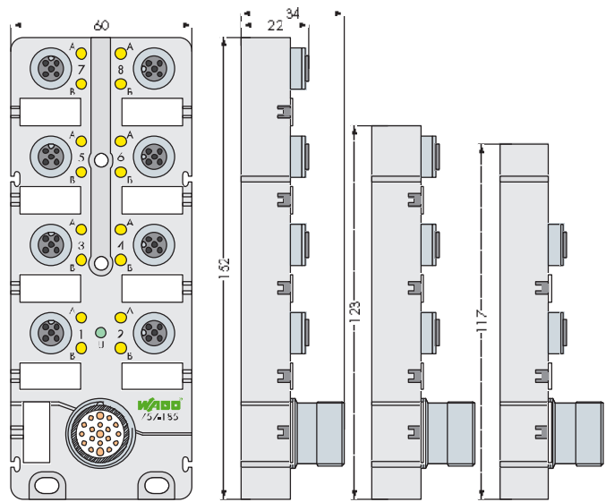
8-гнездовой
