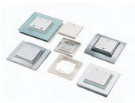
Радиопередатчик, EnOcean easyfit PTM 250
