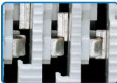
Надежное автоматическое соединение с помощью луженого самоочищающегося скользящего контакта; заземляющий контакт замыкается первым и размыкается последним (серии 750 и 753)
