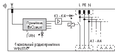
Иллюстрация и структурная схема для 770-629/101-000
