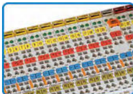
Маркировка зажимных элементов цветными миниатюрными маркерами WSB
