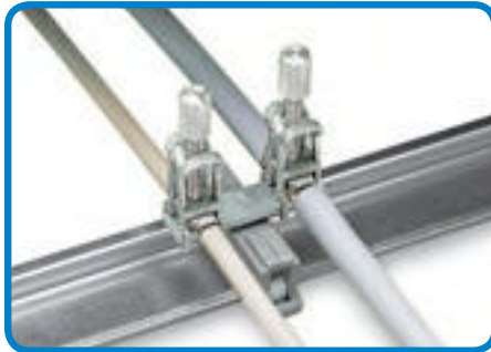
Держатель с заземляющей ножкой 45 мм/1,772 дюйма в длину, шинопровод параллельно рельсу Код 790-114
