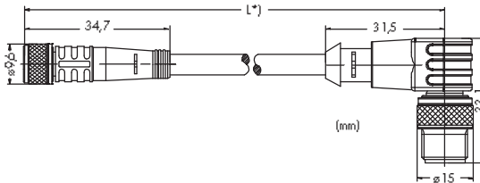
Гнездо M8
