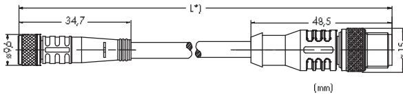
Гнездо M8
