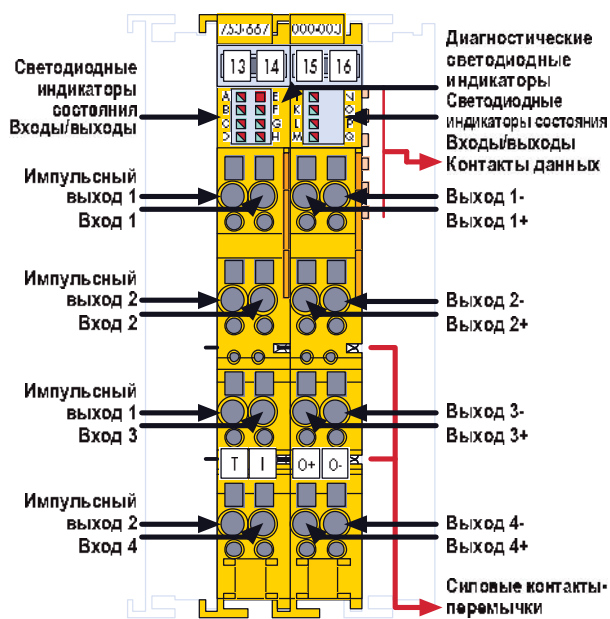
Рис. серии 753/Поставляется без миниатюрных маркеров WSB
