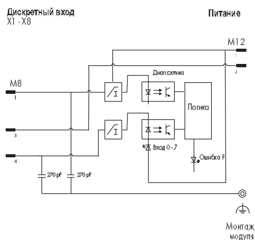
Структурная схема входа
