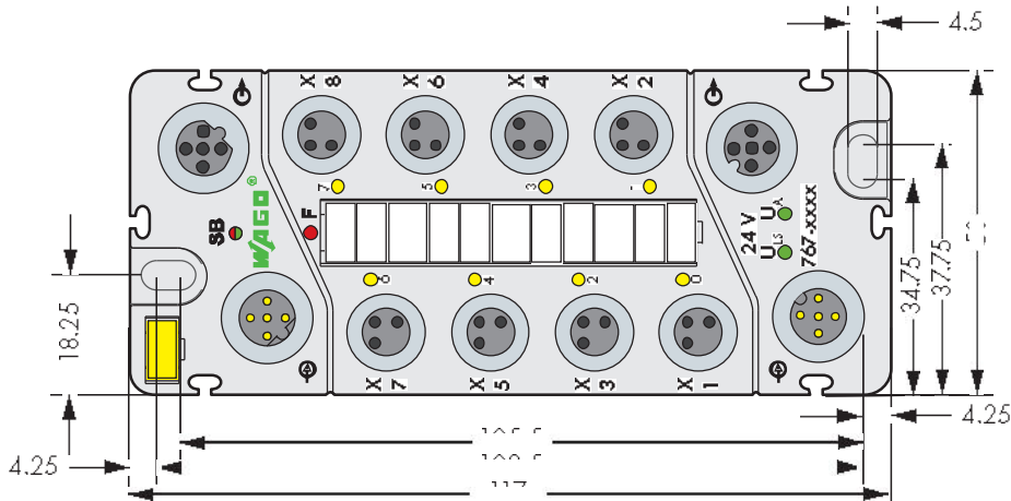
Модуль ввода-вывода
