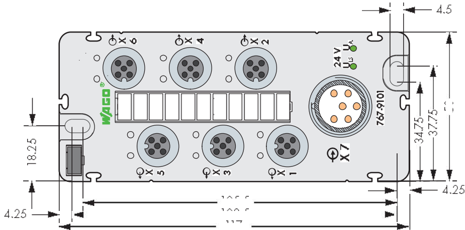
Делитель электропитания
