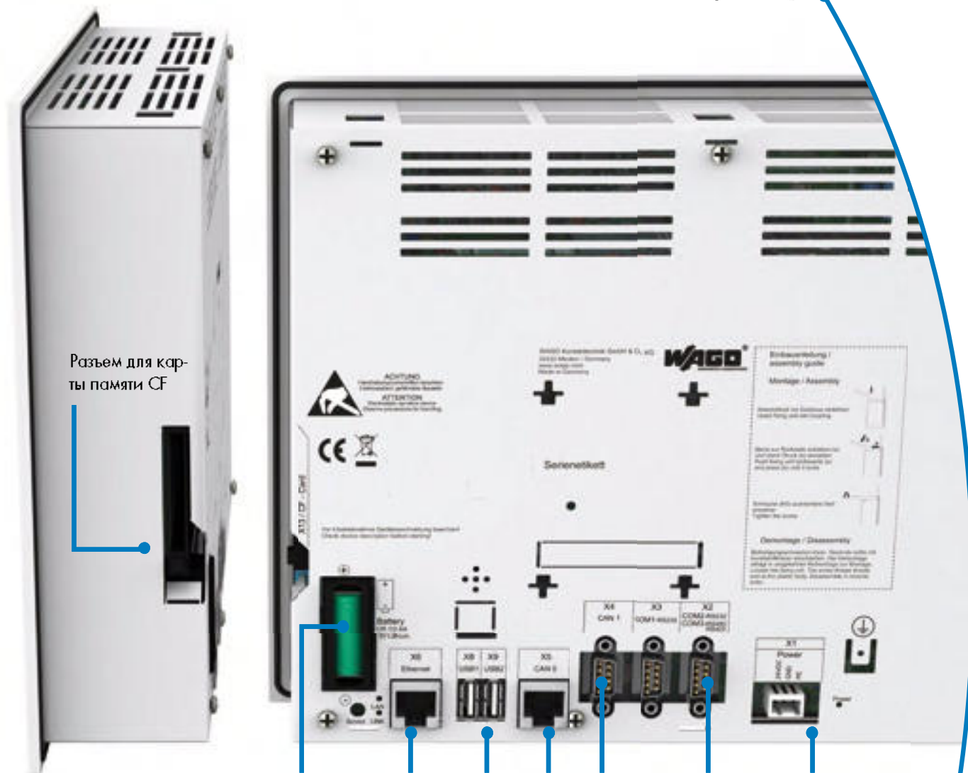
Батарея для буферизации данных в случае нарушения электропитания
