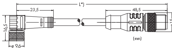
Штекер M12
