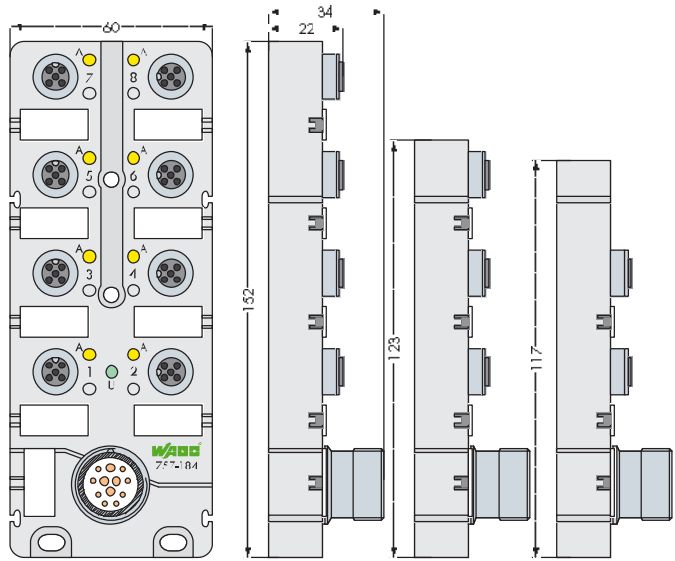
8-гнездовой 6-гнездовой 4-гнездовой
