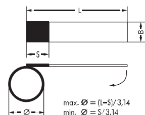
Размеры самоламинирующегося ярлыка
